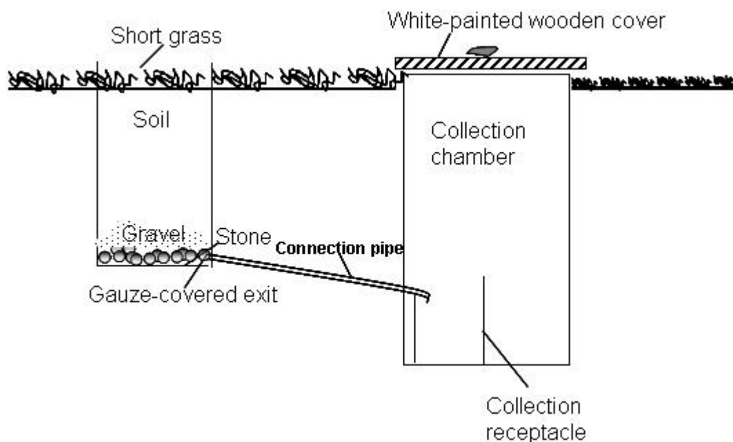
Fig. 28: Evapotranspirometer
