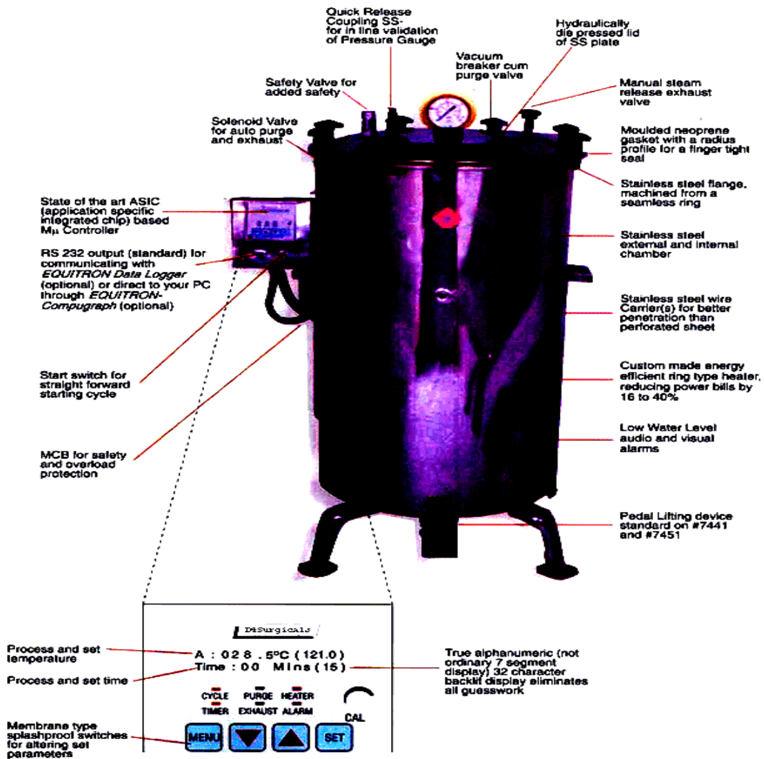
Fig. 3.1: The Autoclave
