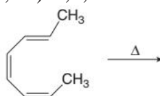
(2E,4Z,6Z)-2,4,6-octatriene
