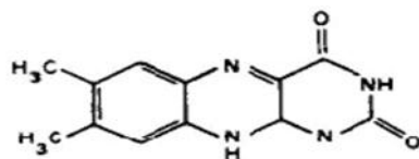
LUMIFLAVIN
