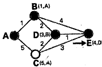
Figure 3.14 (d) Dijkstra Algorithm D
